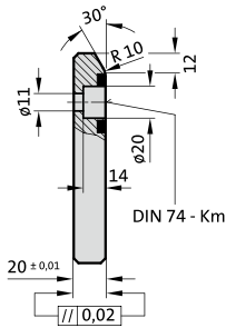
2213. Self-lubricating guide plate, AFNOR/ISO 9183-2 2213. 自润滑导板, AFNOR/ISO 9183-2
