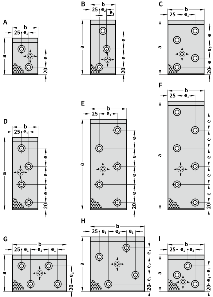
2213. Self-lubricating guide plate, AFNOR/ISO 9183-2 2213. 自润滑导板, AFNOR/ISO 9183-2
